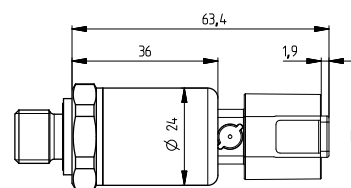
Deutsch DT04-4P
